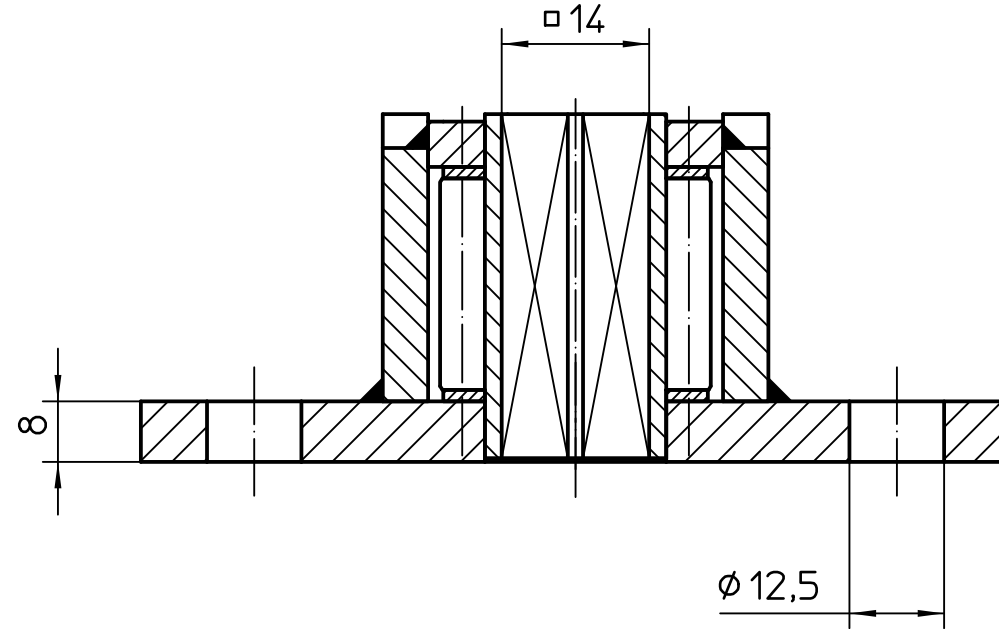
Schnitt B-B
