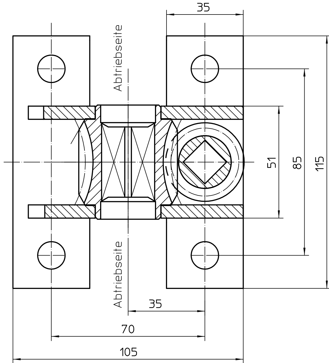
Schnitt A-A
