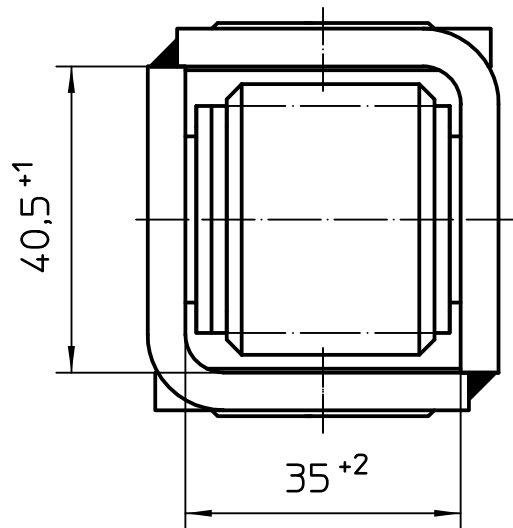
Ansicht "A"
